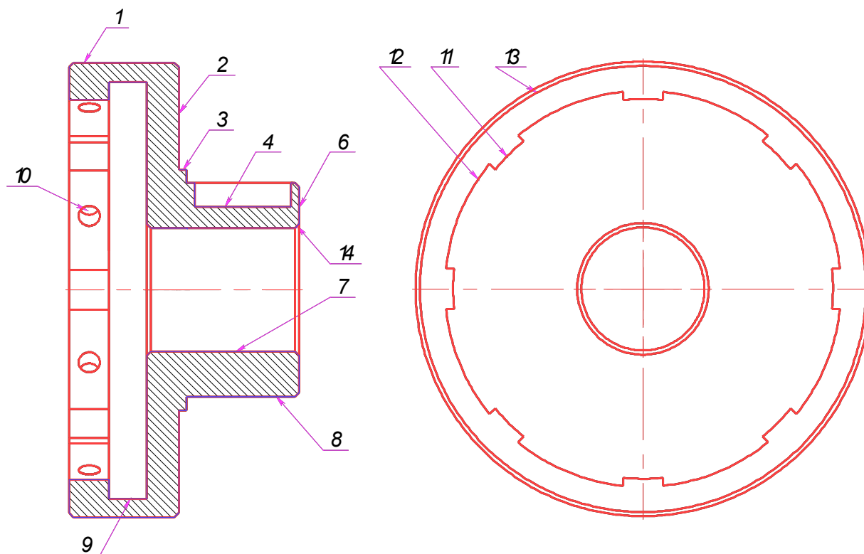
Рисунок 1,2 – Анализ выявления элементарных поверхностей после механической обработки.
