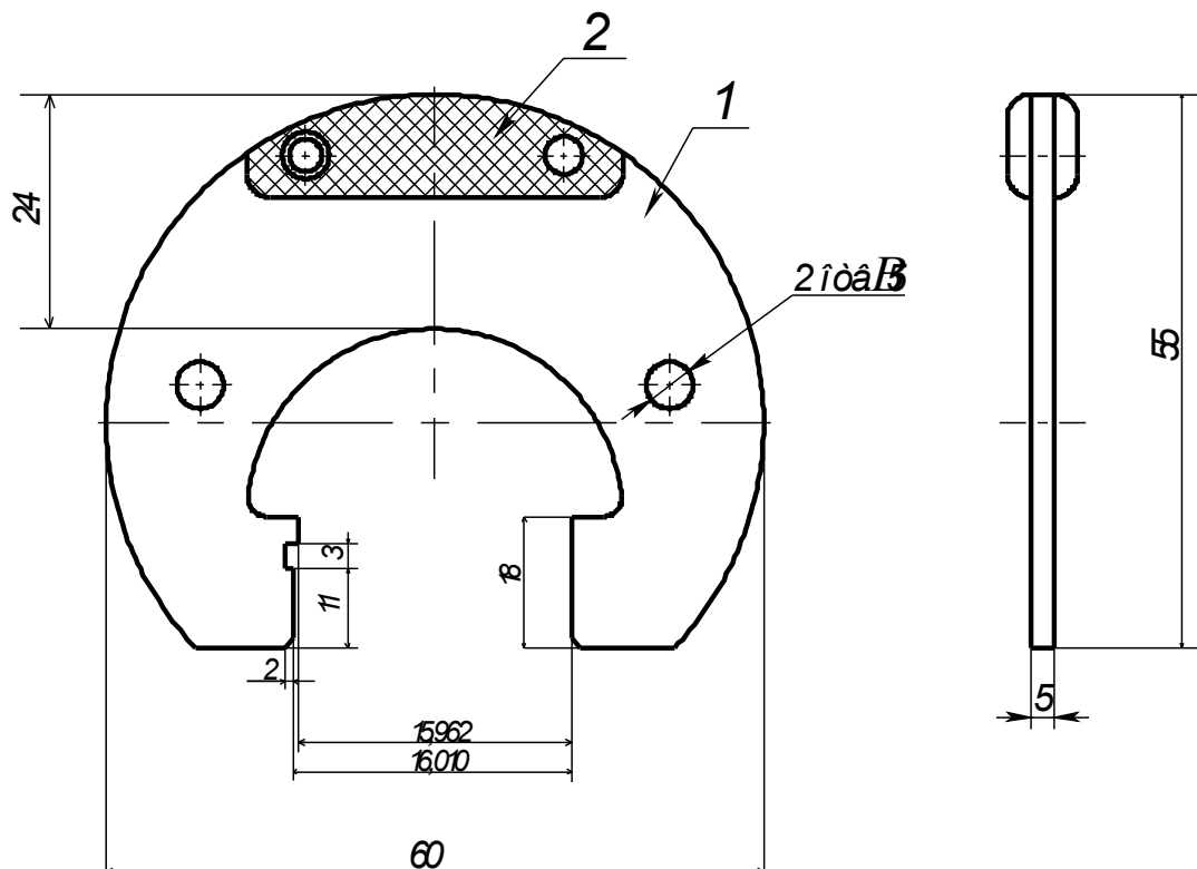
Рис 3.5 – Калибр-скоба для размера Ø16h9).
